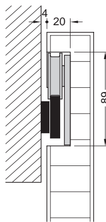
壁面との距離4mm
