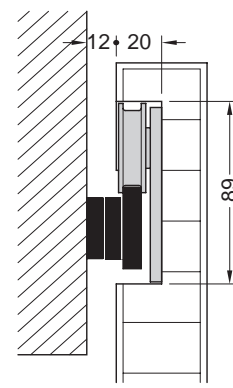
壁面との距離12mm
