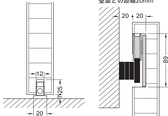
壁面との距離20mm
