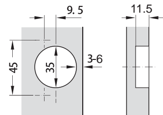
扉加工図
